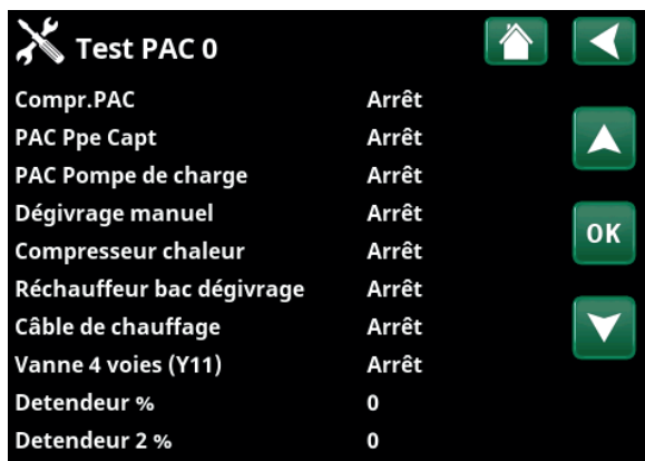
Menu : «Installateur/Service/Test Relais/Test PAC».
